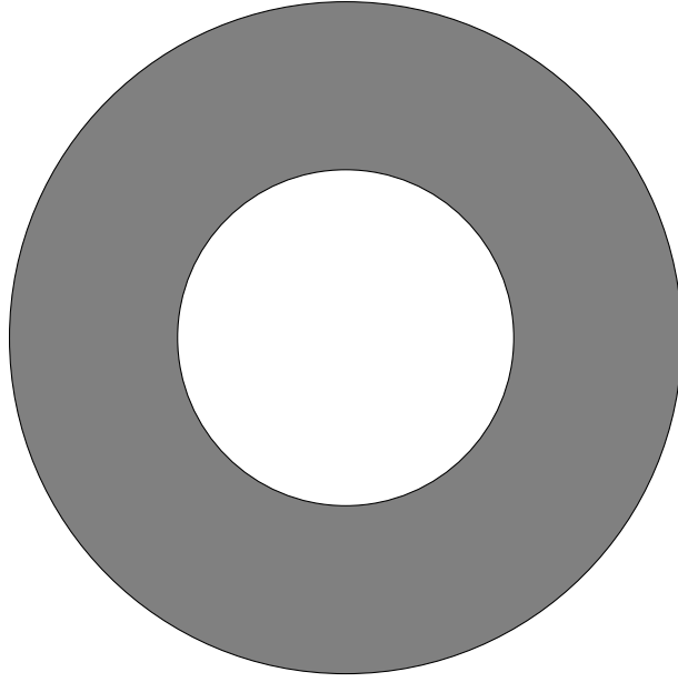
Figura 1.9: Insieme complementare
