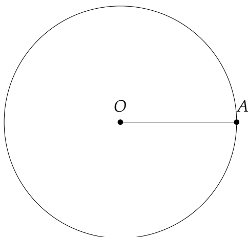
Figura 12.21: Circonferenza
