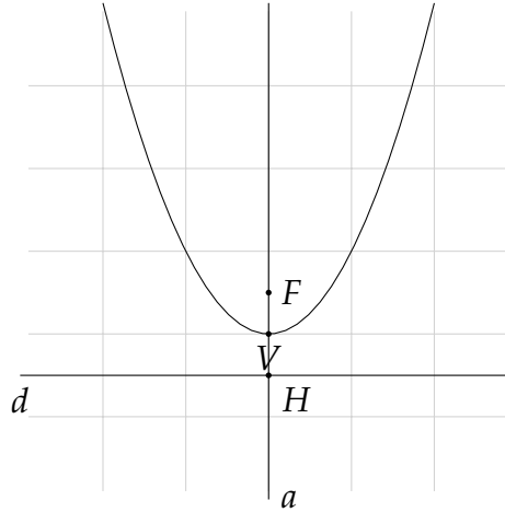
Figura 13.7: Parabola
