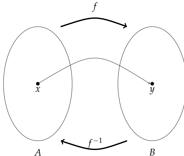
Figura 2.3: Applicazione inversa
