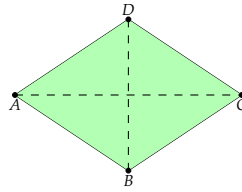
Figura 12.18: Un rombo
