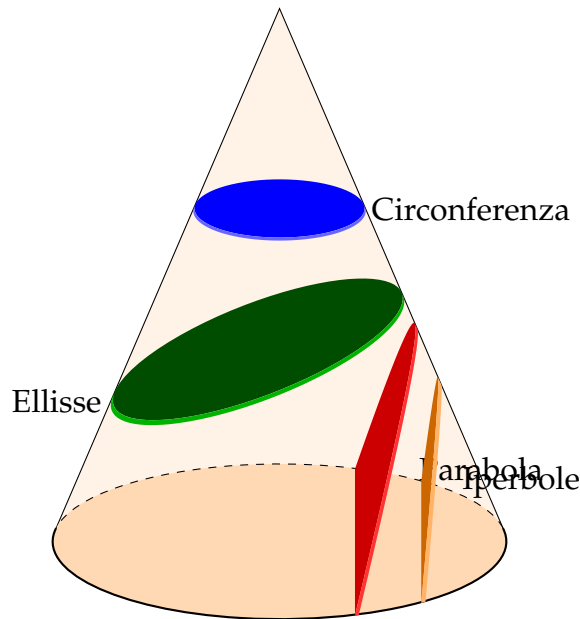
Figura 13.5: Sezione conica
